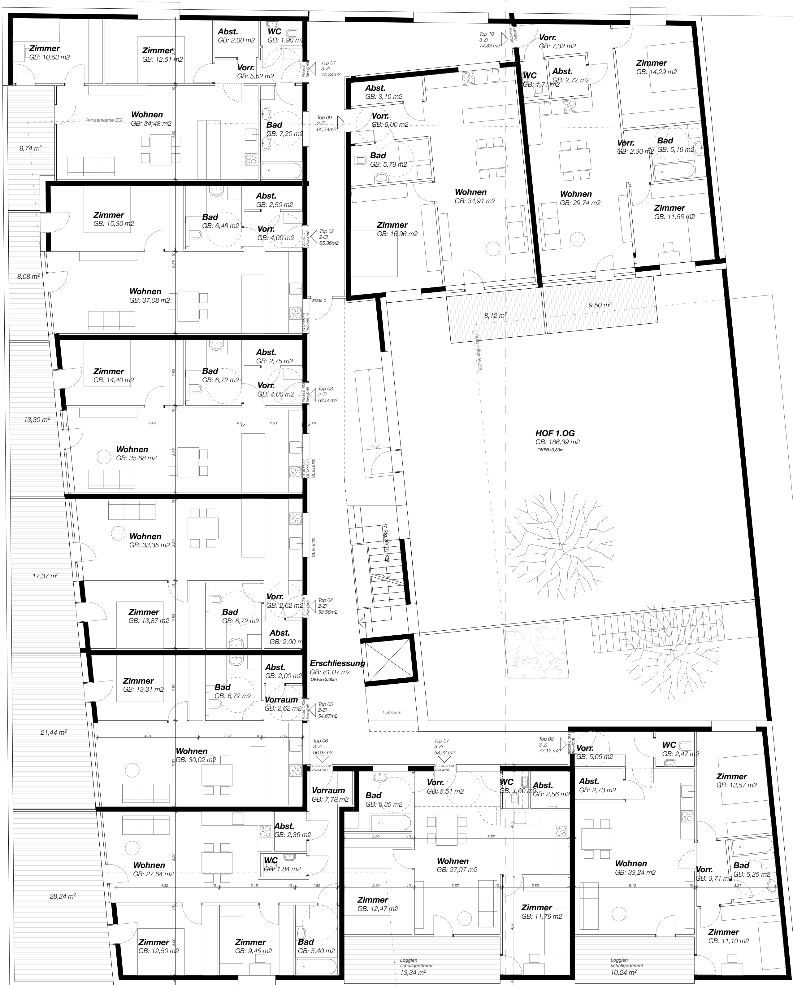
1. OBERGESCHOSS
