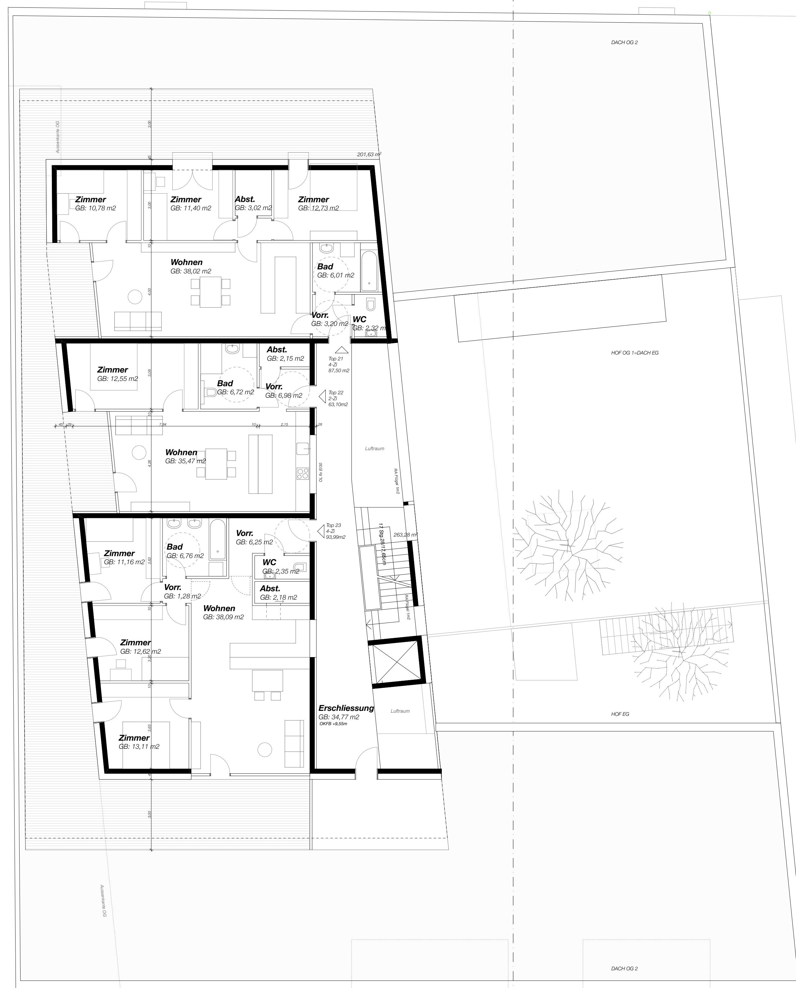
DACHGESCHOSS
