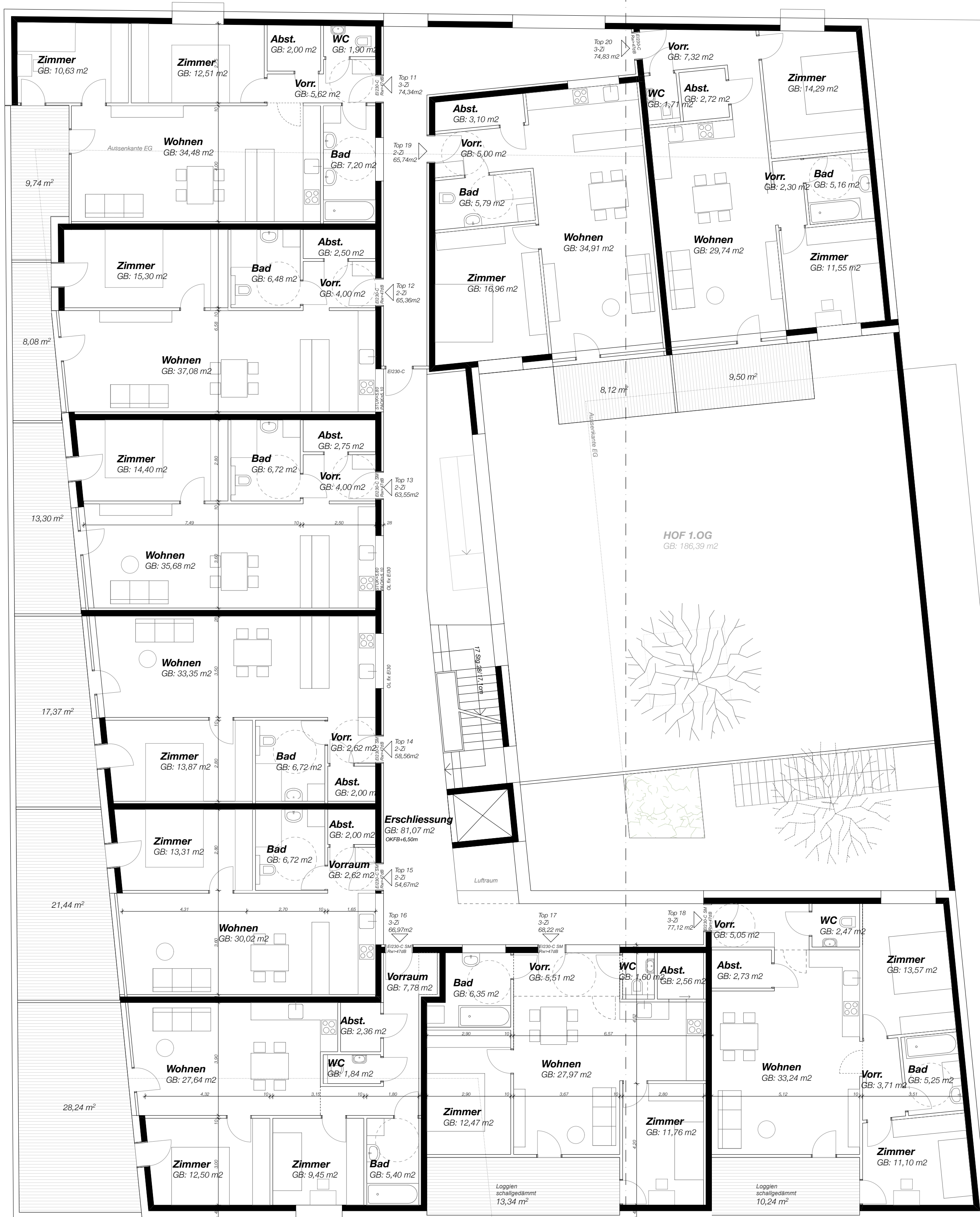
2. OBERGESCHOSS
